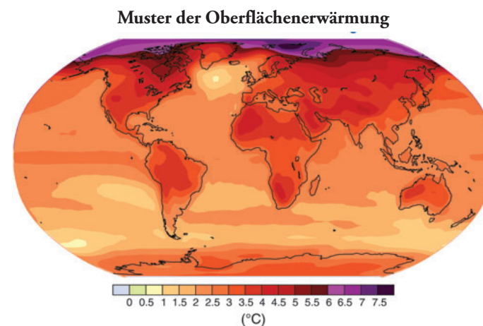
Projizierte Änderungen der Erdoberflächentemperatur für das späte 21. Jahrhundert (2090 - 2099). Die Karte zeigt ein Mittel aus mehreren AOGCM-Projektionen für das A1B SRES-Szenario. Alle Temperaturen sind relativ zum Zeitraum 1980 - 1999, IPCC 2007
